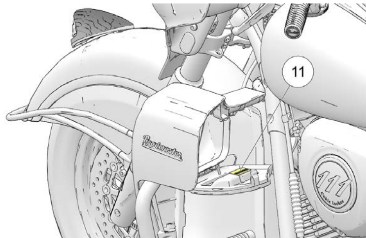
⑪ Capaciteitslabels voor het handschoenenkastje in de onderkuip
